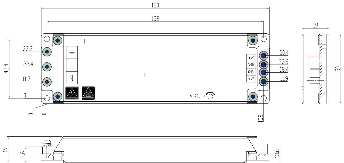
外形尺寸及安装孔——端子坐标图
